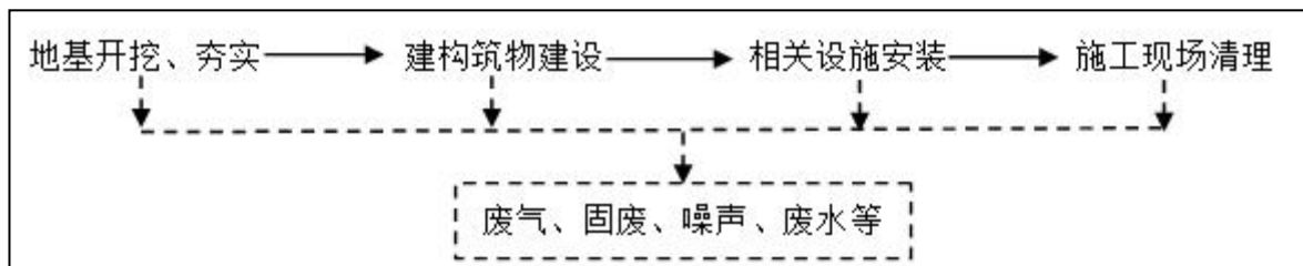
图 2.2-1 施工期工艺流程及产污节点图
